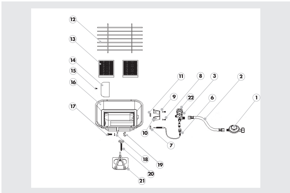
Abb. 4: Explosionszeichnung
